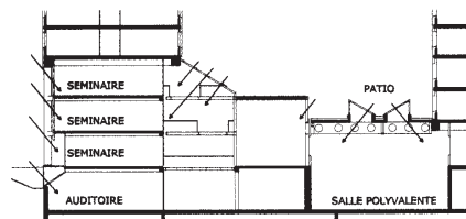
Coupe sur patio
