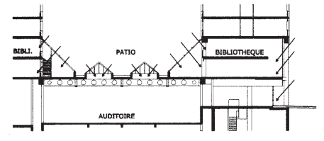
Coupe sur auditoire et bibliothèque
